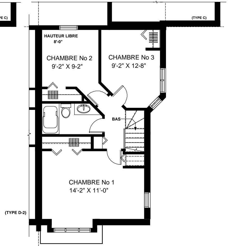
PLAN DE L'ETAGE No 2 SURFACE HABITABLE DE 599 p.c.
