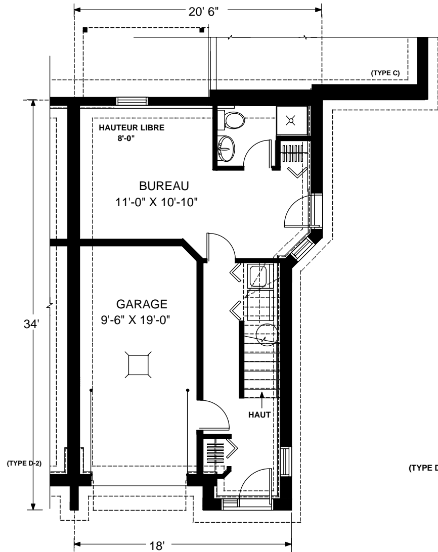
PLAN DU R.D.C. SURFACE HABITABLE DE 425 p.c. SURFACE DU GARAGE DE 218 p.c.
